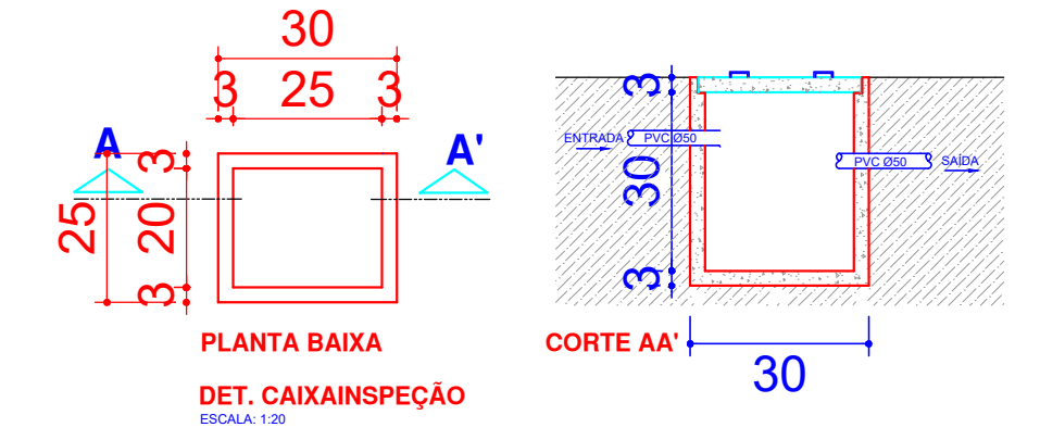
PLANTA BAIXA - HIDRÁULICA
